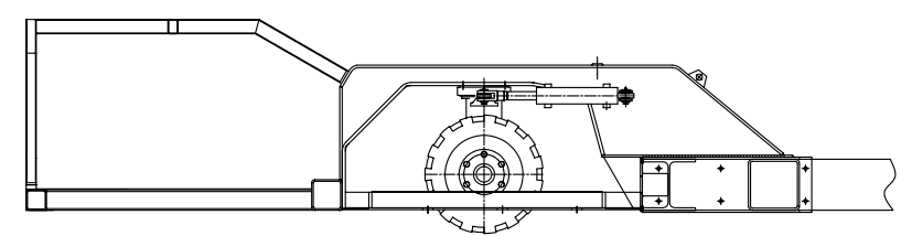
Vista da A (lato motore)
